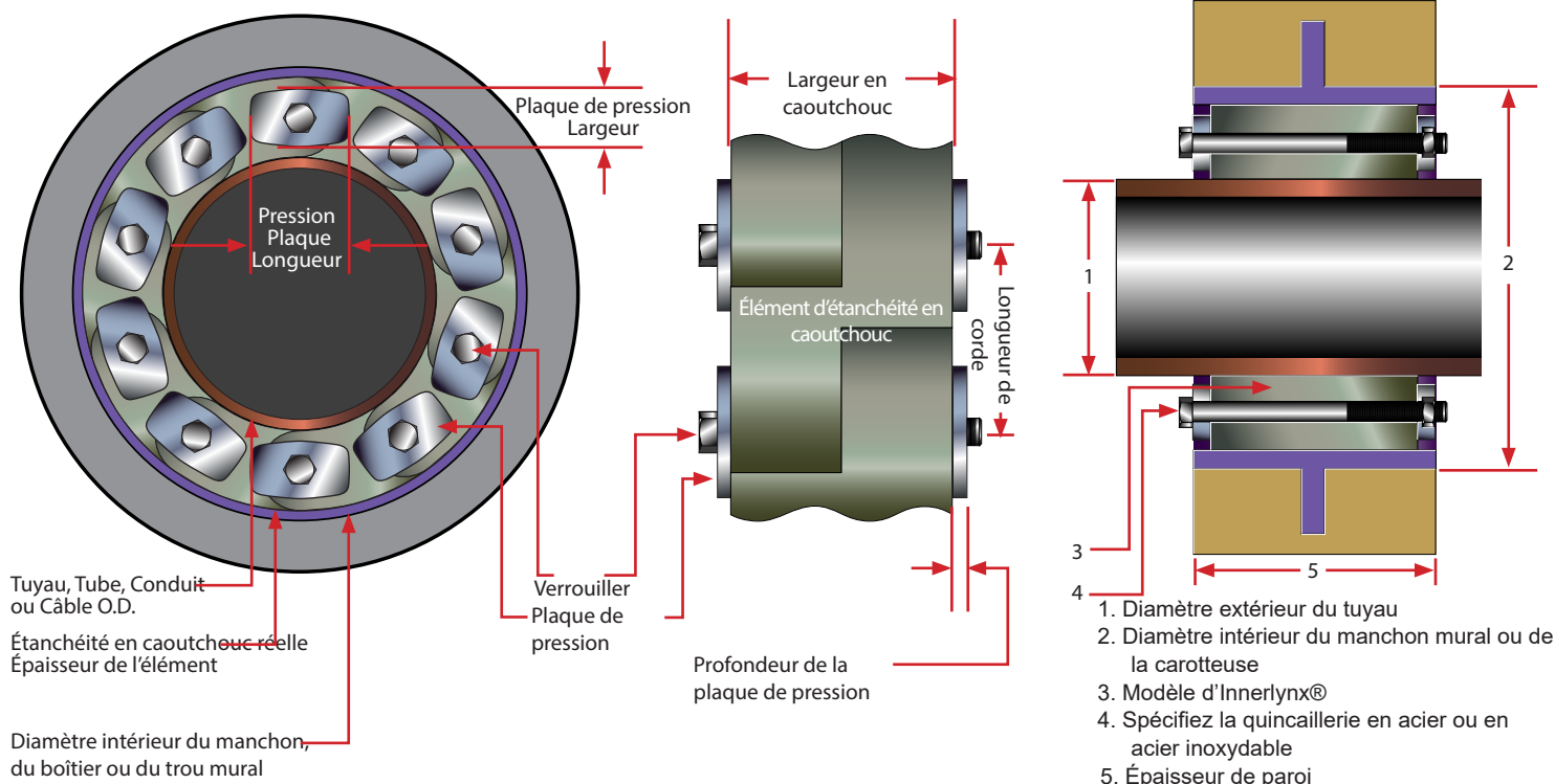
Assemblage Innerlynx® Vue de côté/coupe
