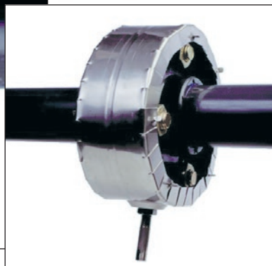
Escudo protector de acero inoxidable con drenaje
