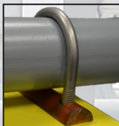
UBolt-Cote® HT con almohadilla de soporte para tubo Atlas® HT Máxima temperatura operativa: 302° F
